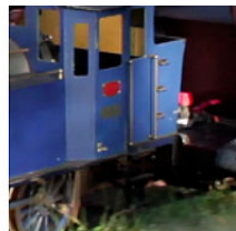
4:4:4
